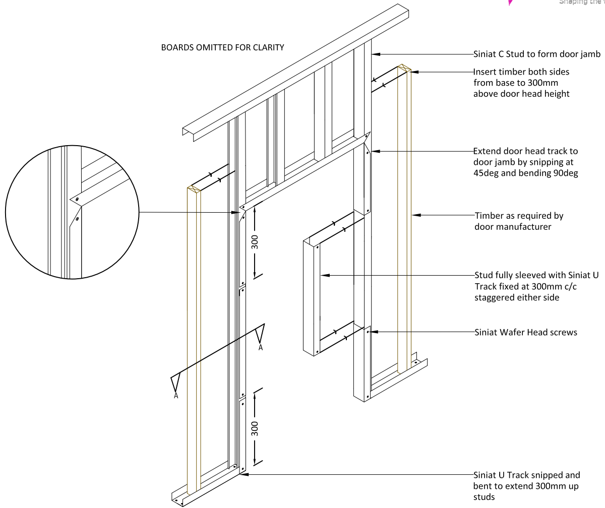
DOOR JAMB ARRANGEMENT
